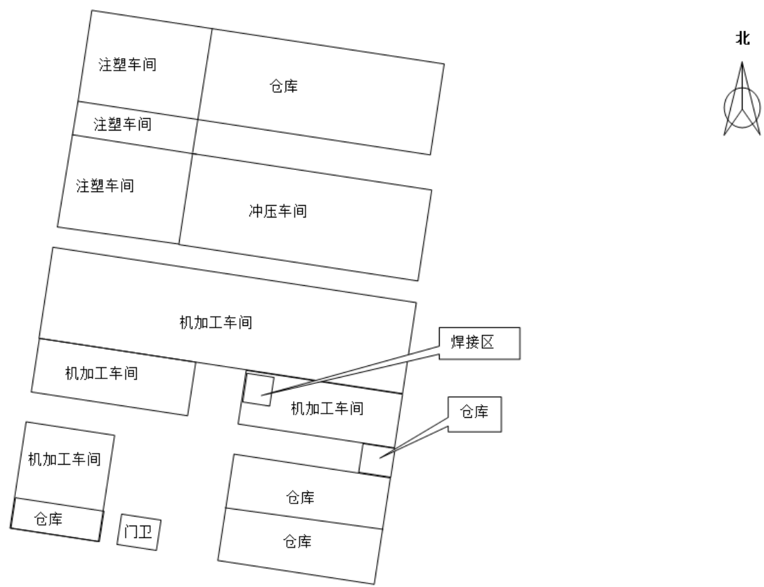
图 3-2 厂区一层平面布置图
