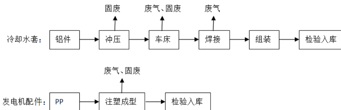
图 3-3 本项目生产工艺流程图
