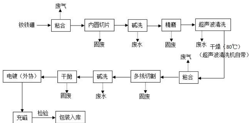
图 3-3 本项目生产工艺流程图
