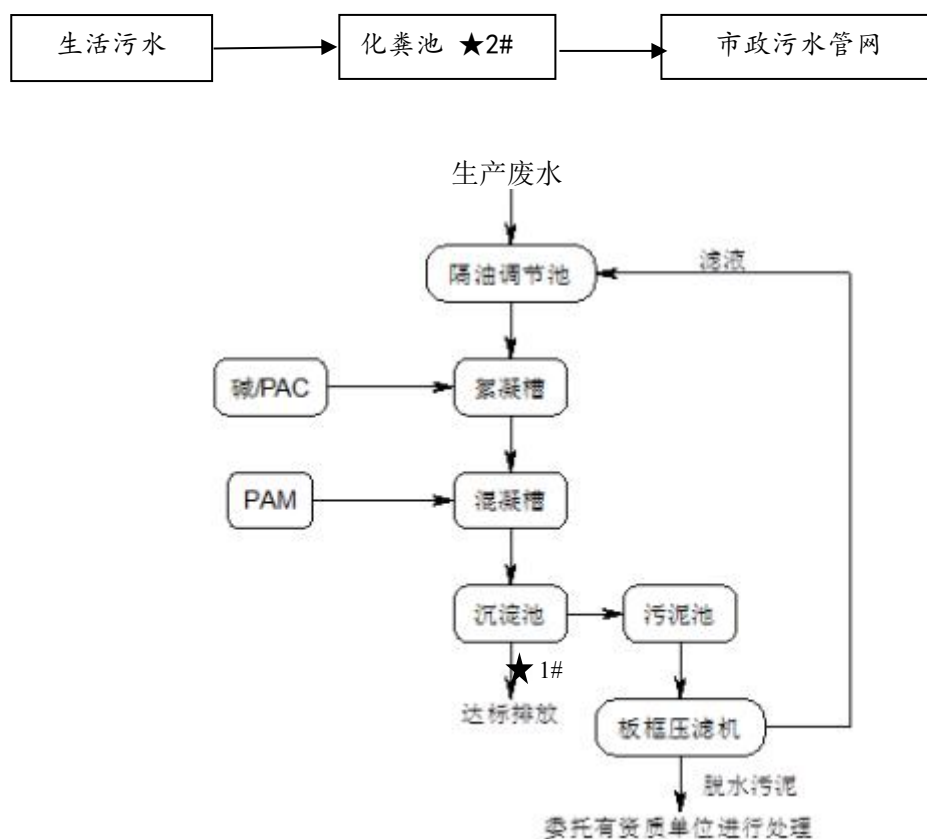
图 4-1 废水处理工艺流程图
