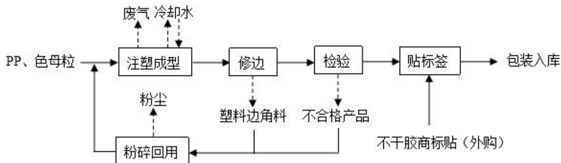
图 3-3 本项目生产工艺流程图
