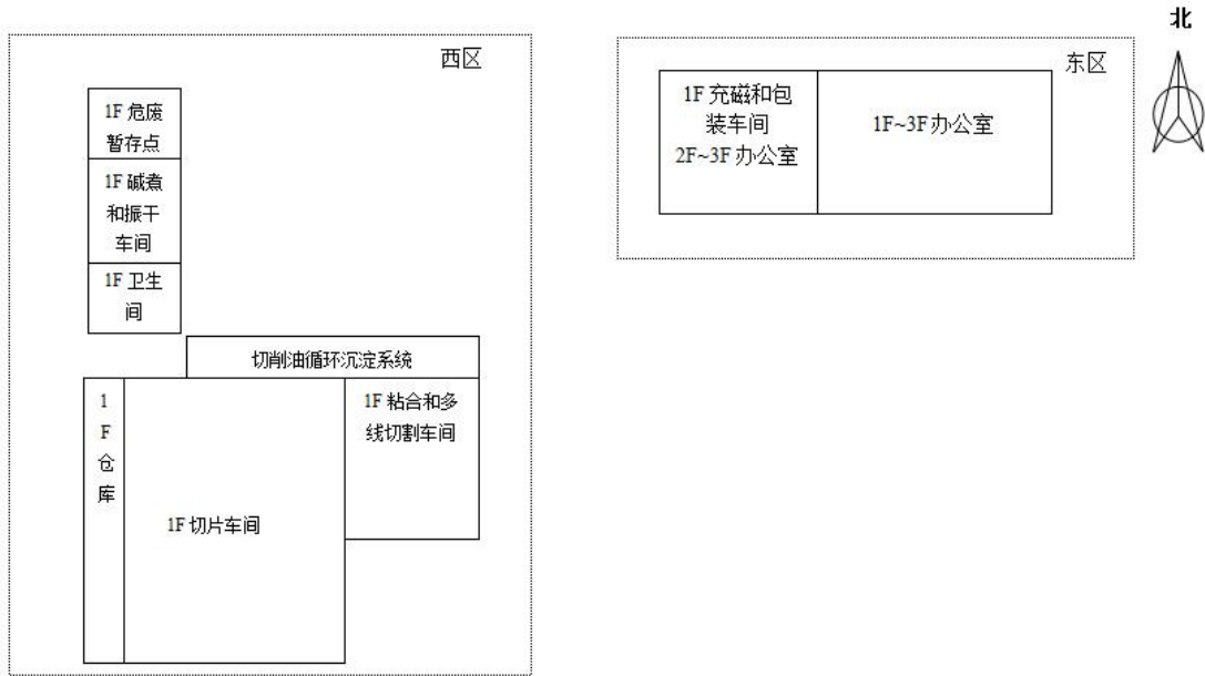
图 3-2 厂区平面布置图
