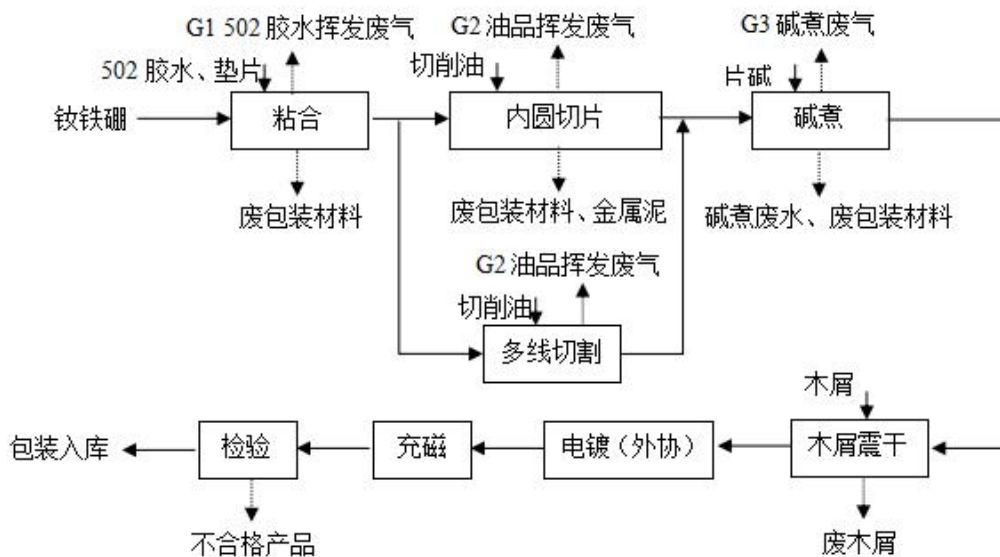
图 3-3 磁钢生产工艺及产污环节示意图
