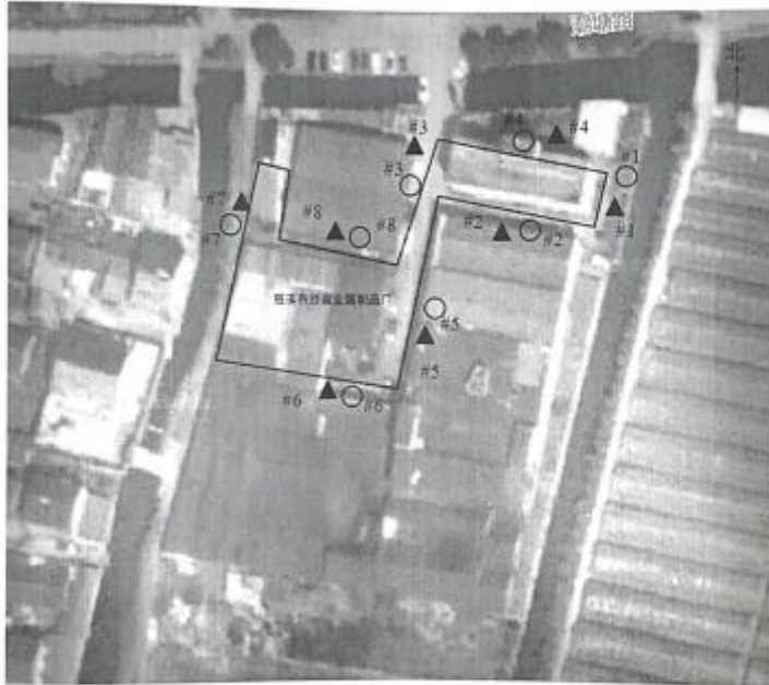
图 2: 测点示意图
