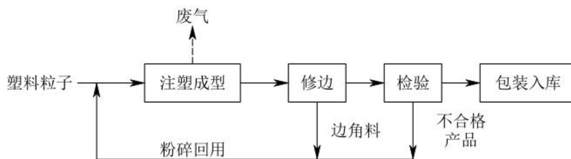
图 3-3 本项目生产工艺流程图
