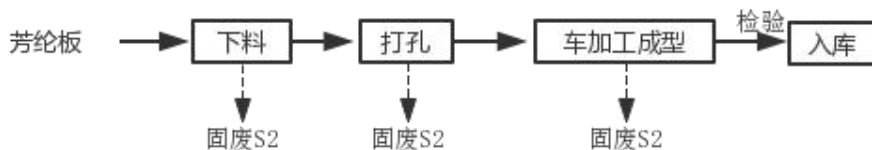
图 2-2 芳纶密封件生产工艺流程及产污节点图
