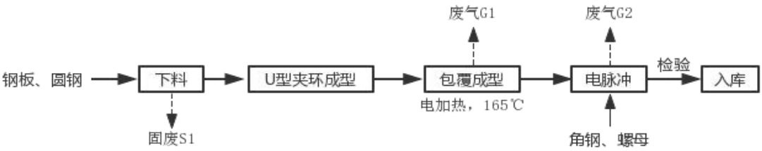
图 2-1 U 型夹环生产工艺流程及产污节点图
