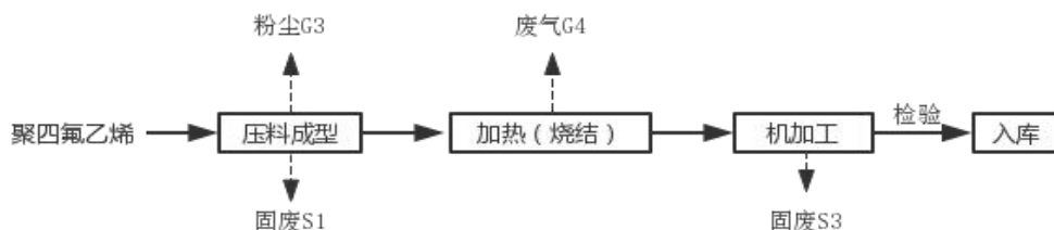
图 2-3 聚四氟乙烯密封件生产工艺流程及产污节点图
