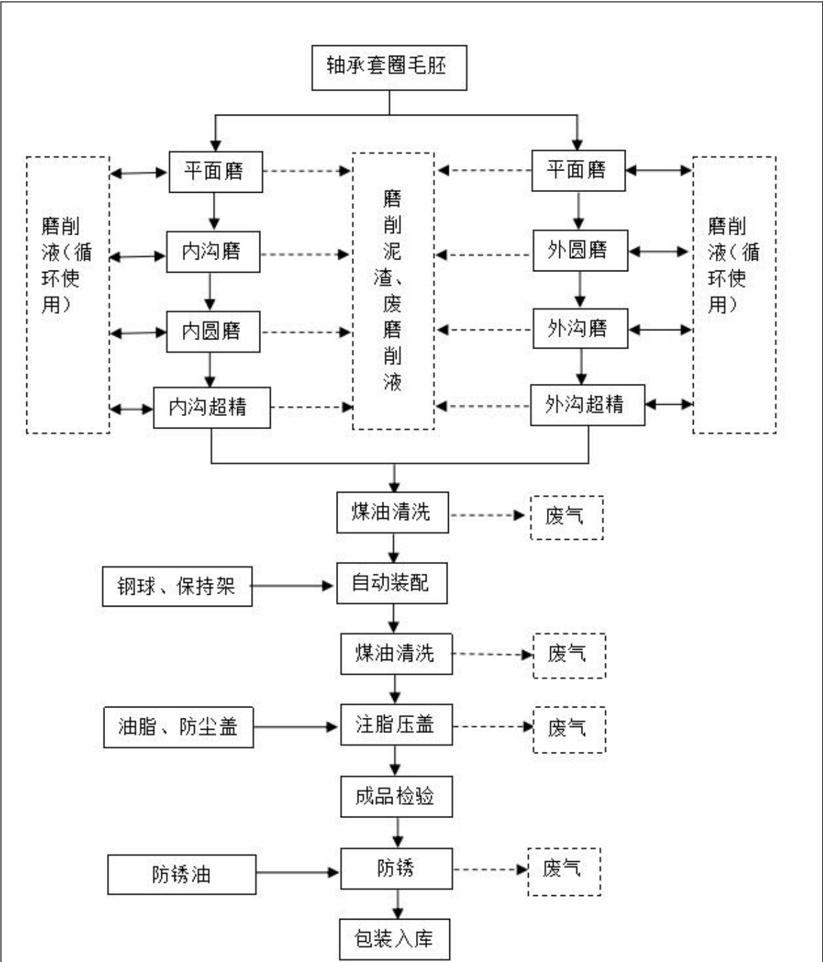
图 2-1 轴承生产工艺流程及产污节点图
